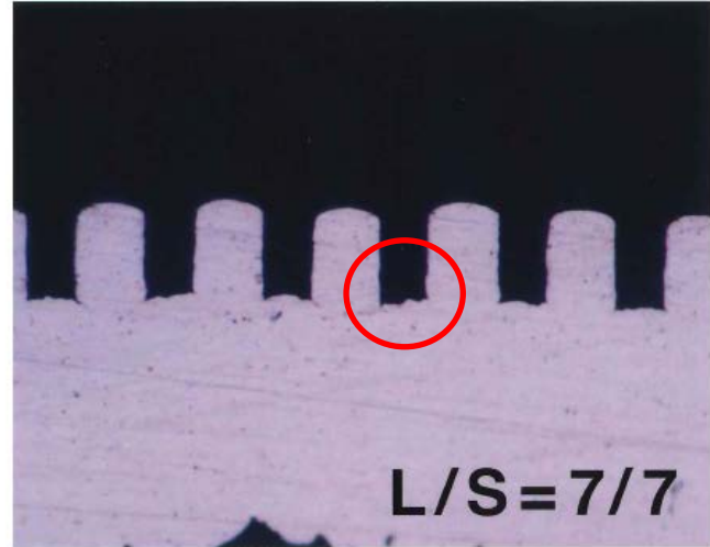
断面写真 (パターンめっき後)
