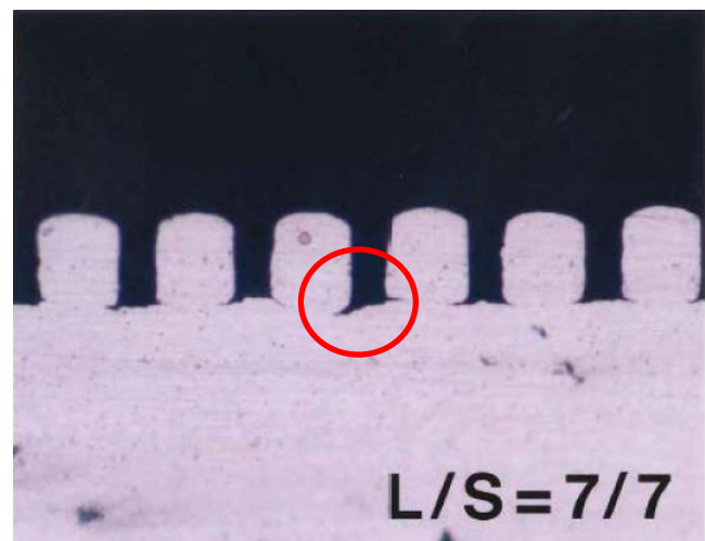
断面写真 (一流体现像処理後パターンめっき)
